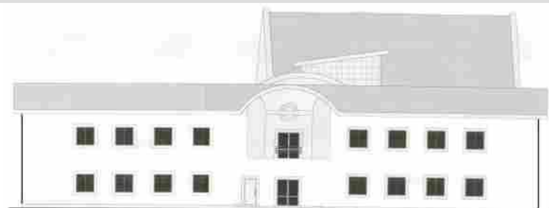
ELEWACJA OD UL. OGRODOWEJ skala 1:100
